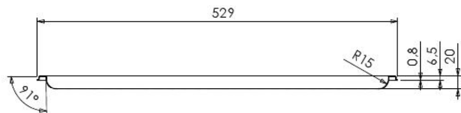
SEZIONE A-A
