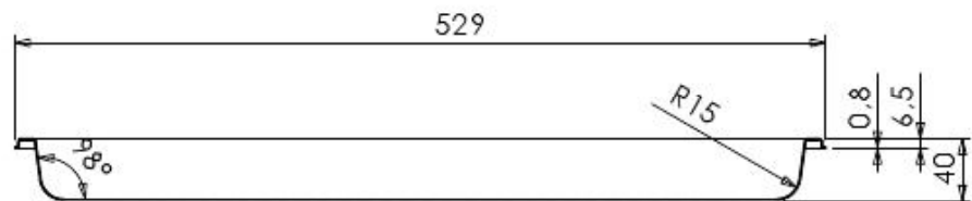
SEZIONE A-A
